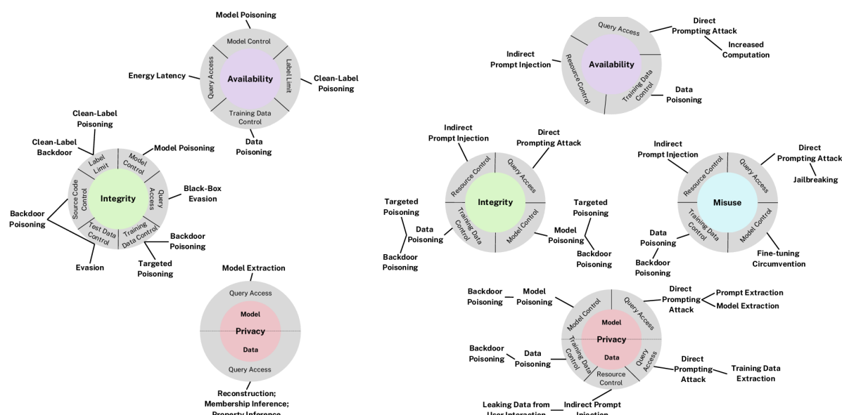
Figure 9 – Attaques sur l'IA prédictive (à gauche) et sur l'IA générative (à droite) d'après le référentiel NIST.AI.100-2e2025
