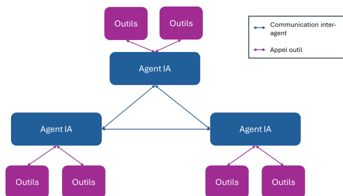
Figure 16 – Exemple de système multi-agent décentralisé
