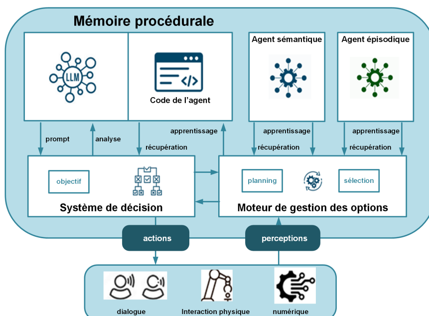
Figure 14 – Exemple de système agentique
