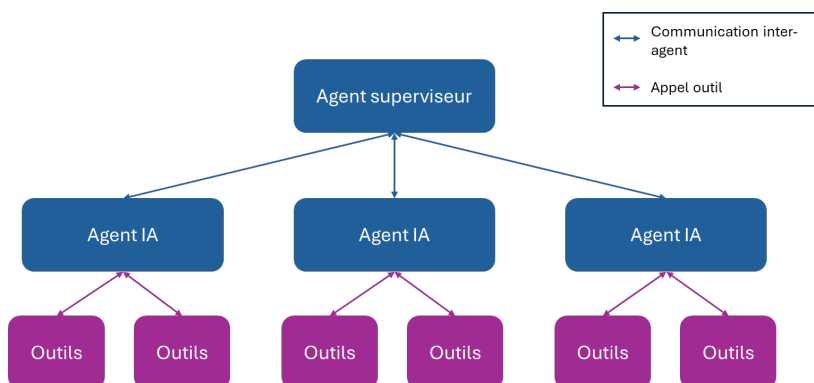
Figure 15 – Exemple de système multi-agent centralisé
